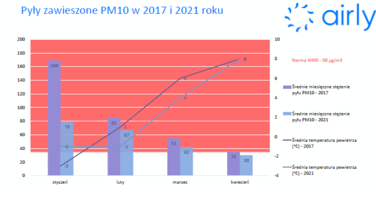
Wykres nr 12. Poziom zanieczyszczeń PM 10
