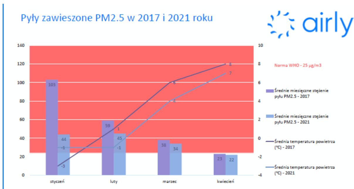
Wykres nr 11. Poziom zanieczyszczeń PM 2,5
