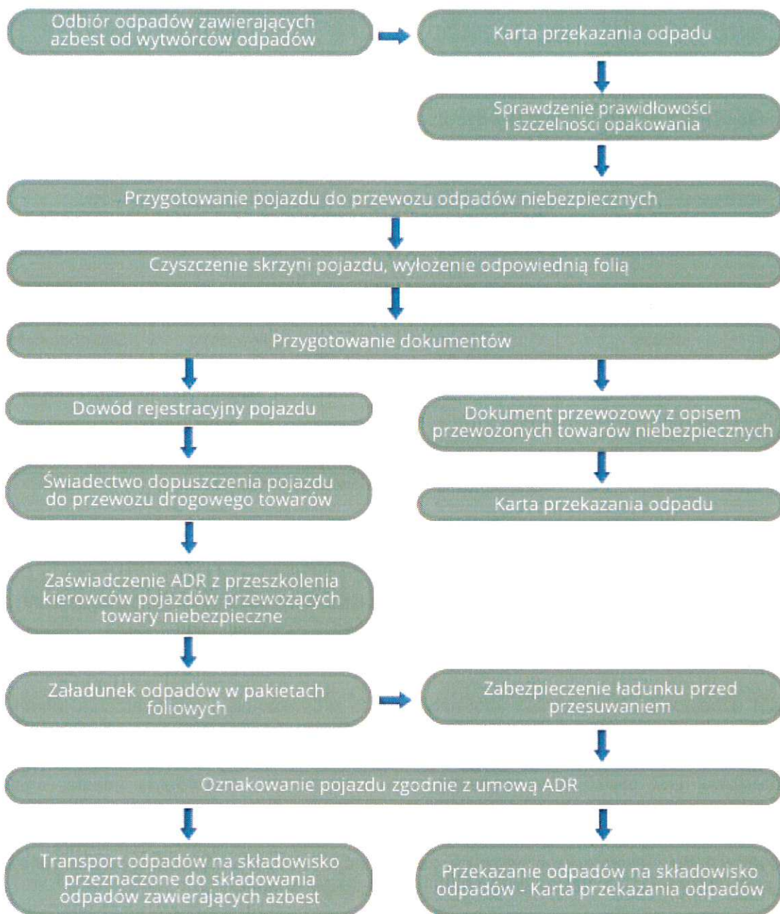
Rysunek 8. Schemat procedury dotyczącej przygotowania i transportu odpadów niebezpiecznych zawierających azbest.
