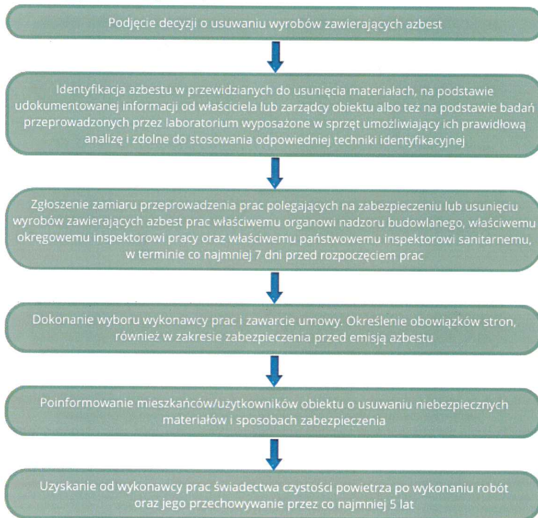
Rysunek 5. Schemat procedury dotyczącej obowiązków i postępowania właścicieli i zarządców przy usuwaniu wyrobów zawierających azbest z obiektów i terenów zlokalizowanych na terenie Gminy Zielonki.
